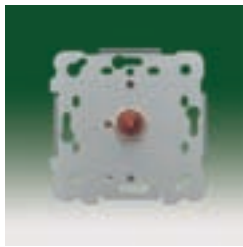
Переключатель поворотный 18596 10А 250V~ Упак. 1 4 позиции, 3 цепи Суппорт для крепления на винтах (без фиксаторов)
